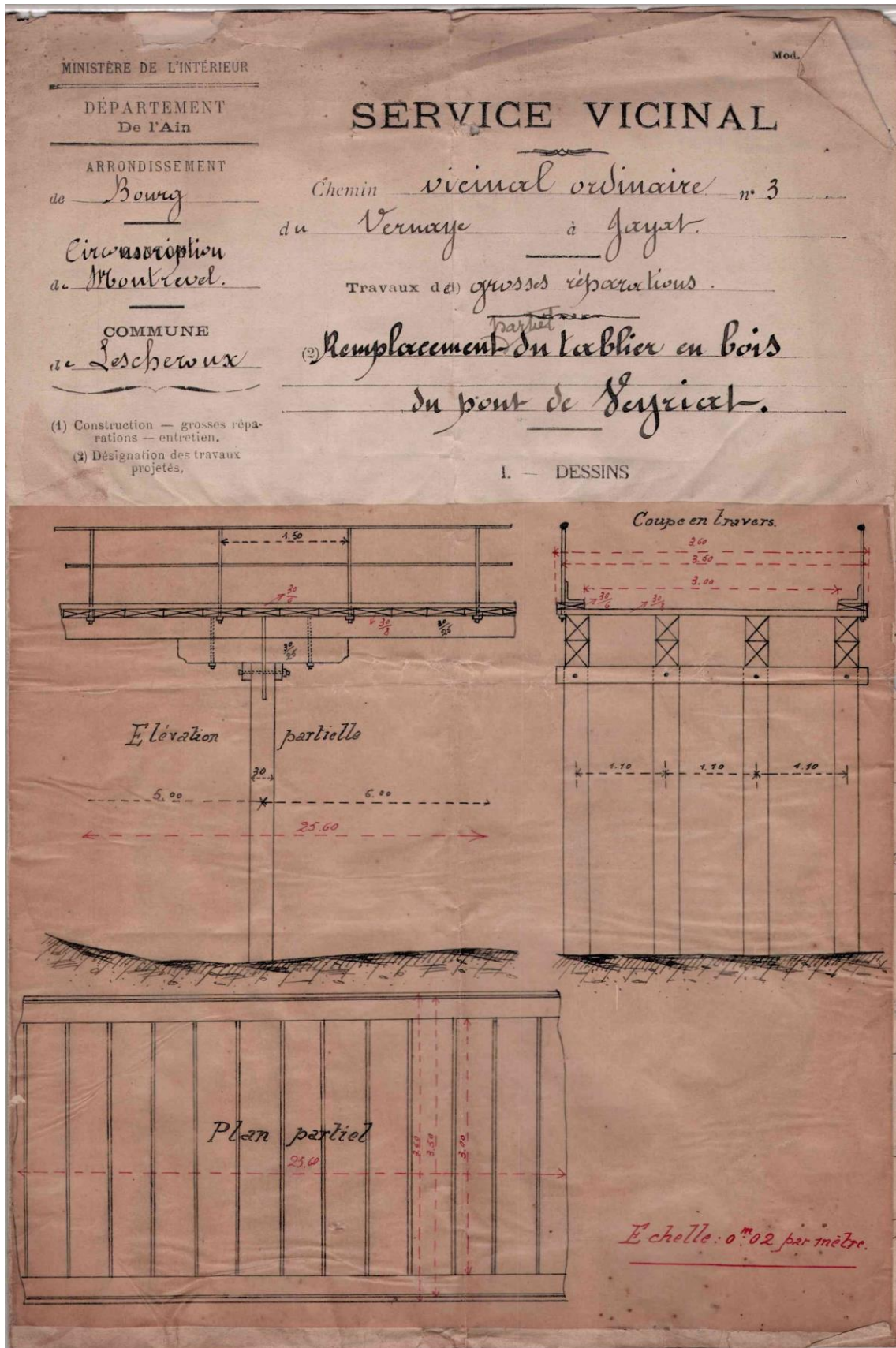
Figure 3 - Plan du Pont de Veyriat, remplacement du tablier, 106 (1917)
