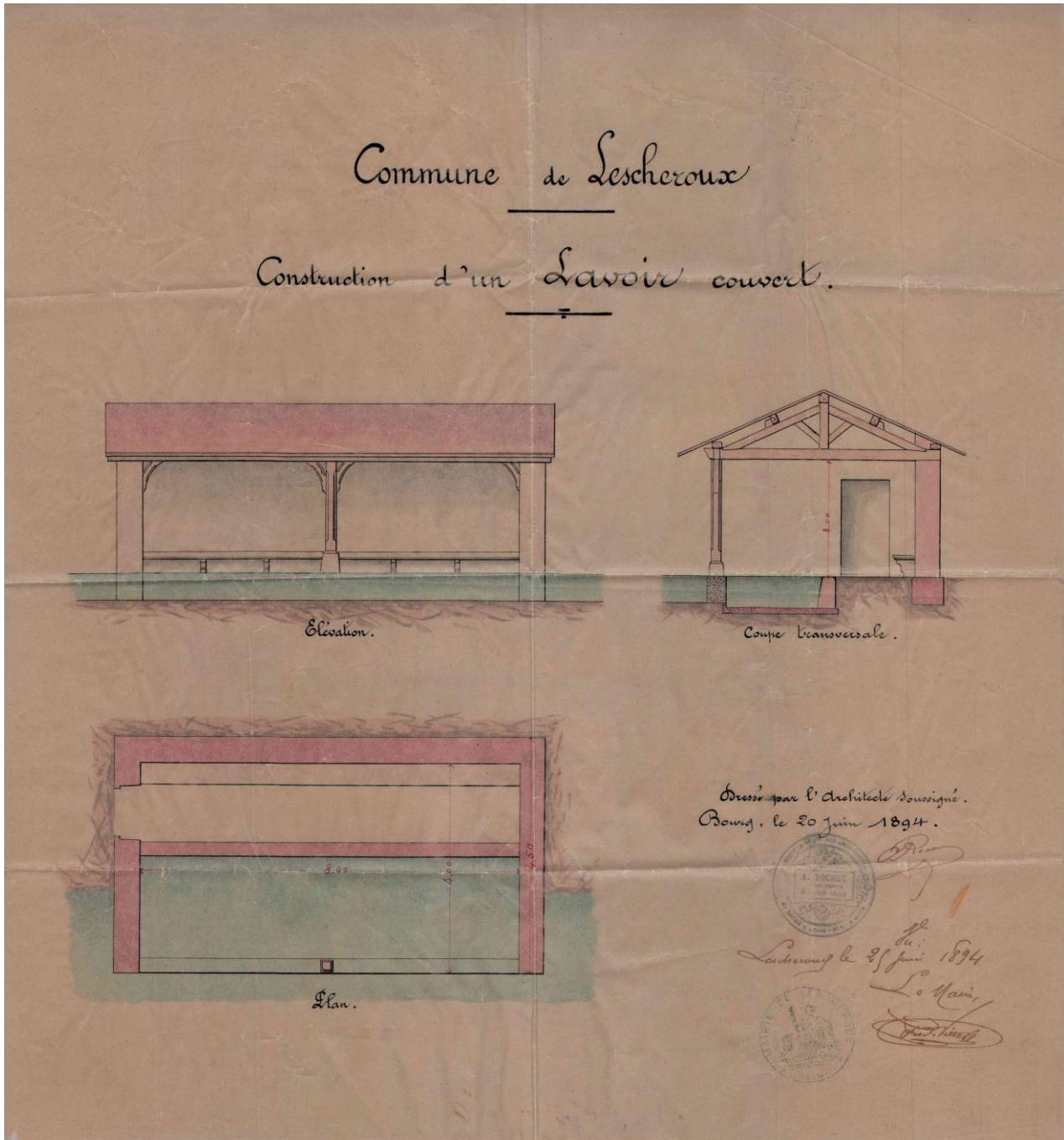
Figure 1 - Plan d'un lavoir, 1M1 (1894)
