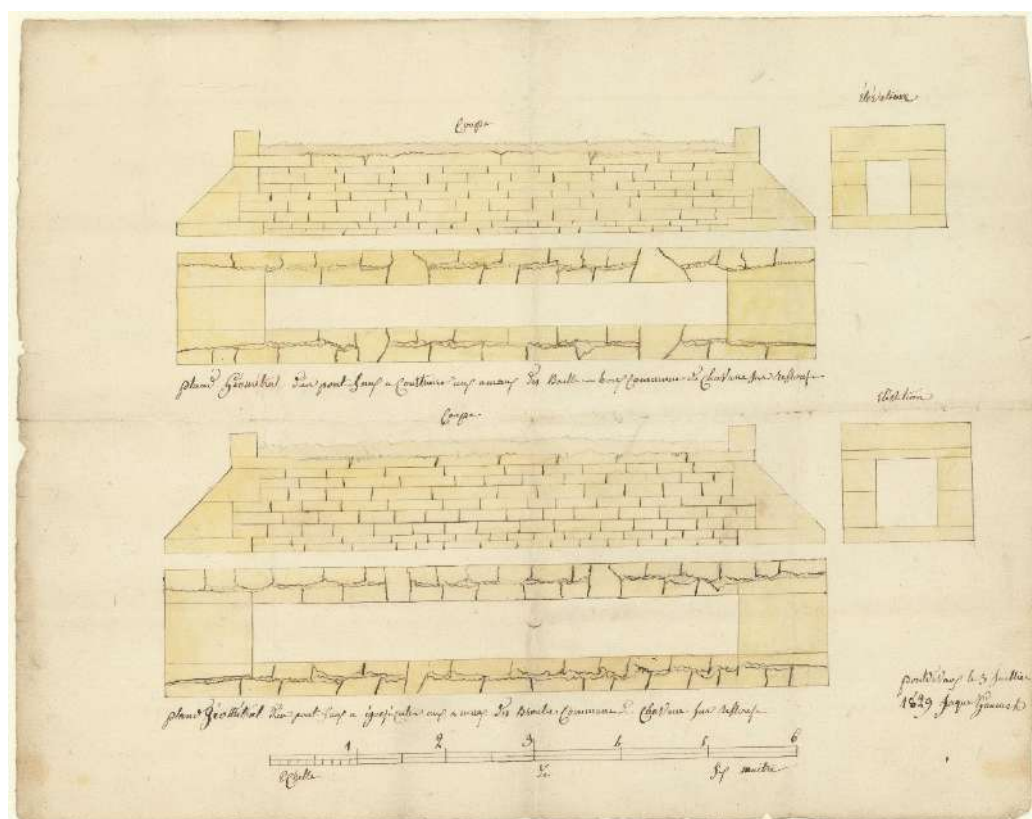
Figure 22 – Plan pour la construction de deux ponts sur le bief des Broubes et au hameau de Bailleboeuf, 105 (1829).
