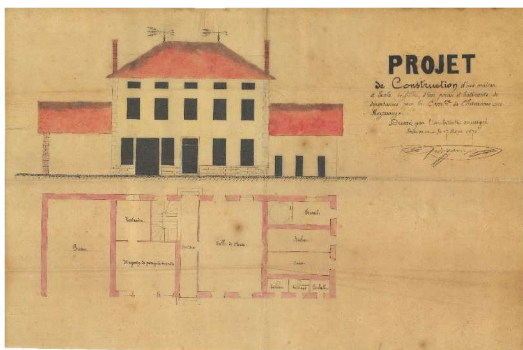
Figure 21 – Plan pour la construction du bâtiment de l'école des filles avec préau et dépendances, 4M2 (1870).
