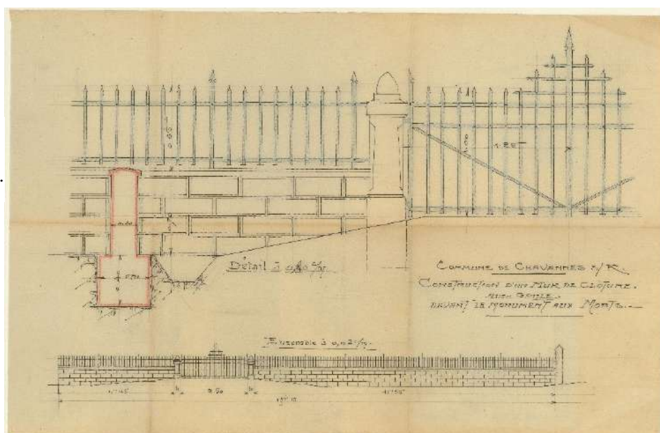
Figure 18 – Plan calque pour la construction d'un mur de clôture avec grille au monument aux morts, 1M2 [1921].
